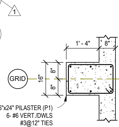
2 S2 DETAIL SCALE: 1/2" = 1'-0"
