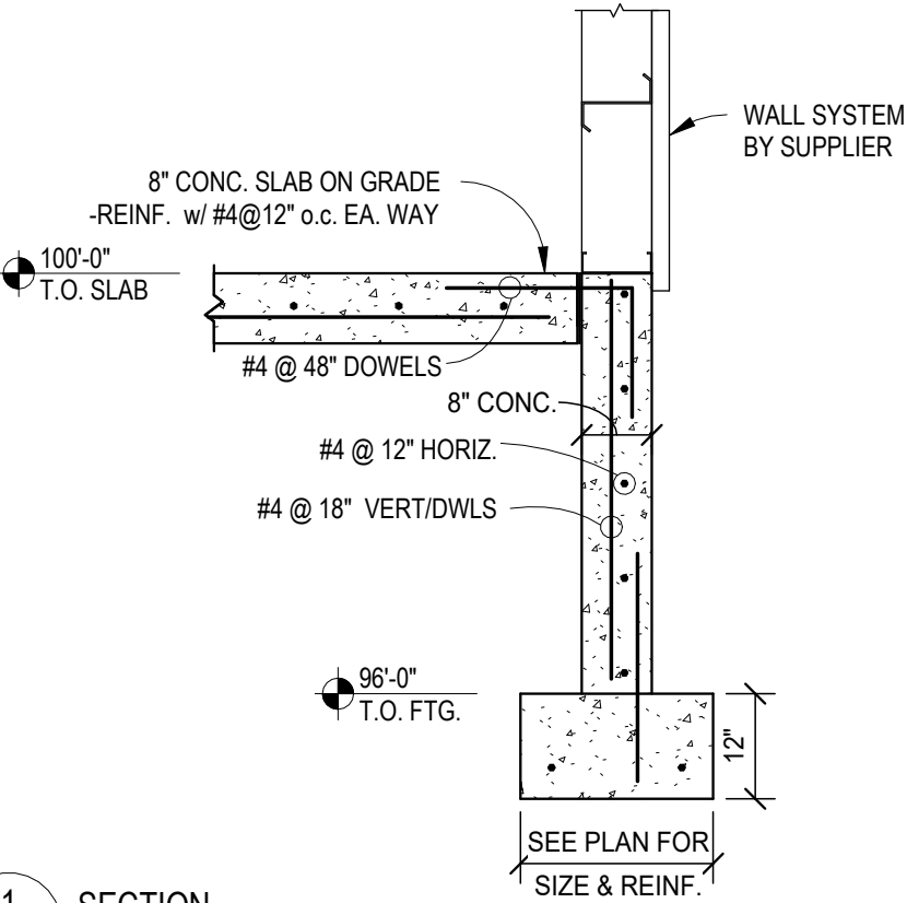
1 S2 SECTION SCALE: 1/2" = 1'-0"
